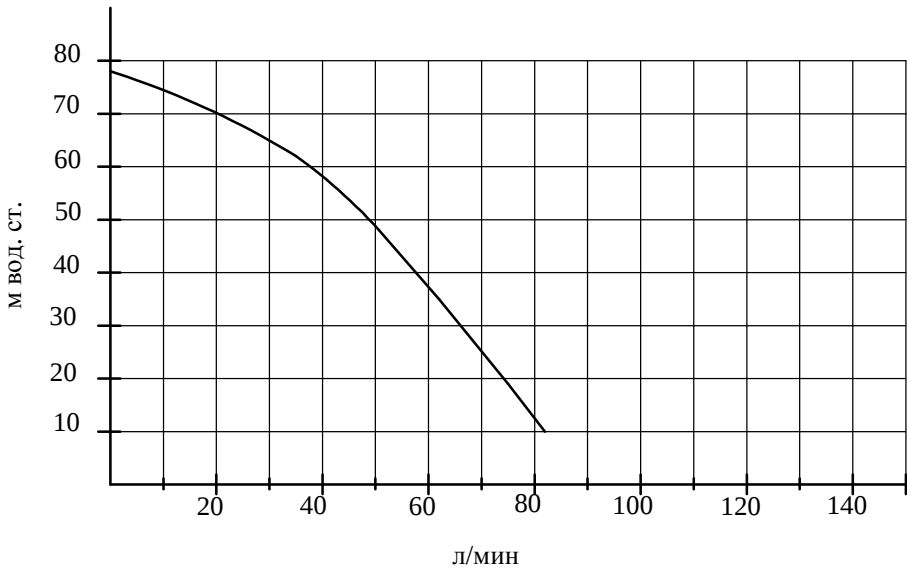
Рисунок 1 – Гидравлическая кривая МПОВ исполнение 00, 01, 02
