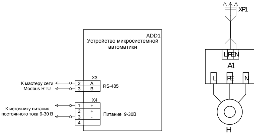
Схема подключения для исполнения 02
